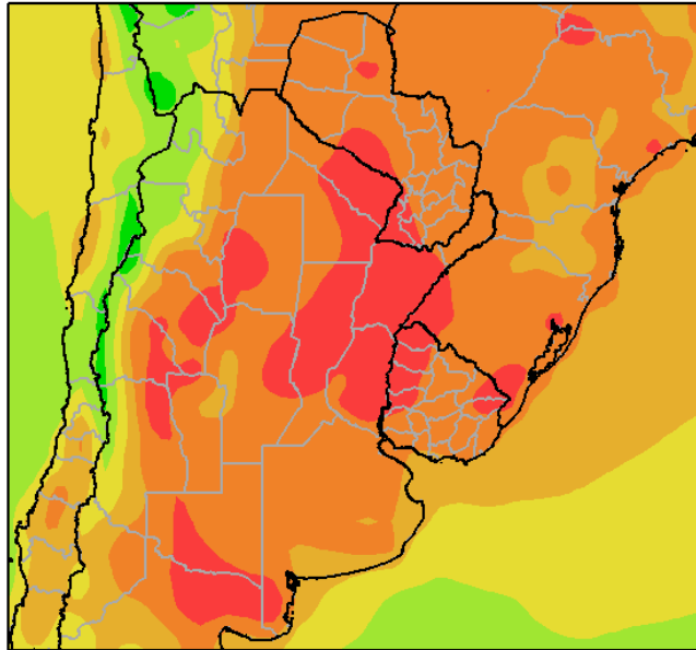
Perspectiva Climática del 23 al 29 de Enero de 2014 Temperatura Maxima (Grados Centigrados)
