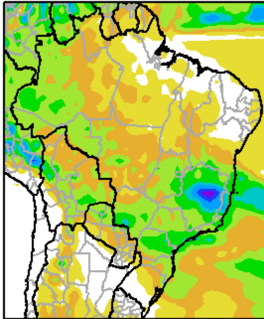
Perspectiva Climática del 3 al 9 de Octubre de 2013 Precipitación Acumulada (mm)
