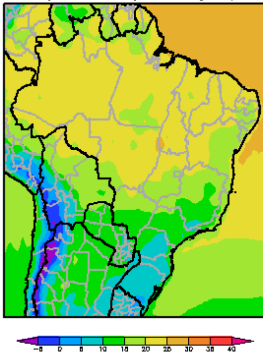
Perspectiva Climática del 3 al 9 de Octubre de 2013 Temperatura Mínima (Grados Centígrados)
