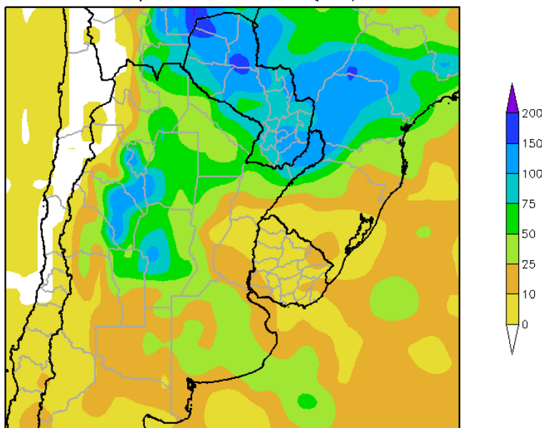
Perspectiva Climática del 10 al 16 de Octubre 2013 Precipitación Acumulada (mm)
