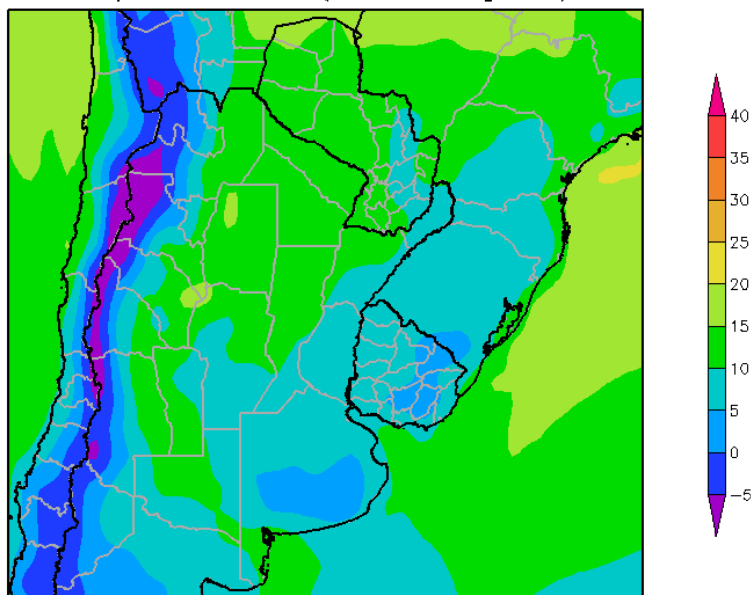
Perspectiva Climática del 3 al 9 de Octubre 2013 Temperatura Mínima (Grados Centígrados)
