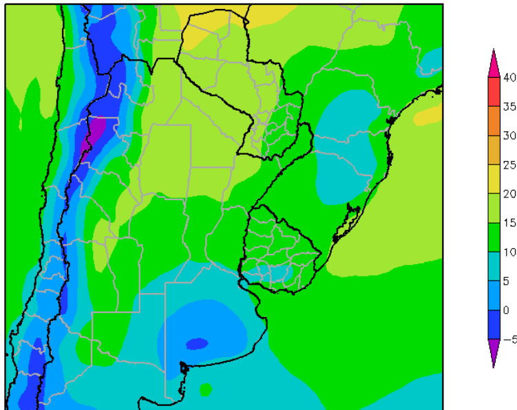
Perspectiva Climática del 10 al 16 de Octubre 2013 Temperatura Mínima (Grados Centígrados)
